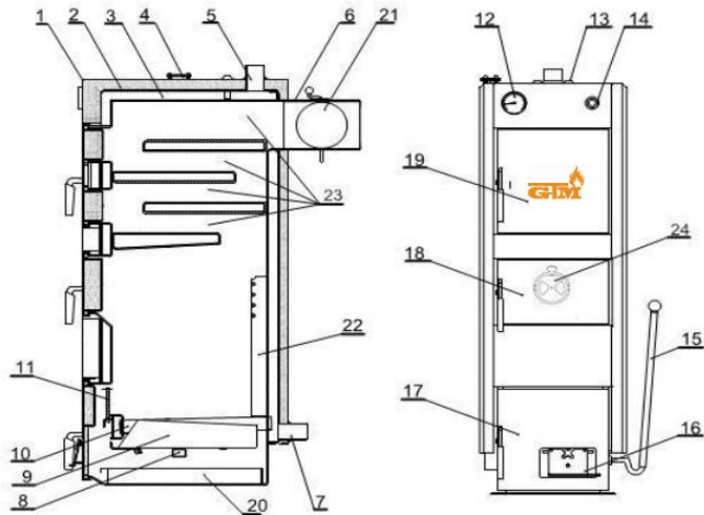
Рисунок 2. Конструкция котла
